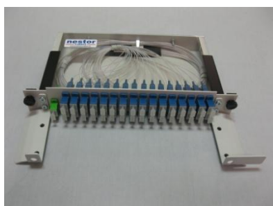
NC-1000 –jaotinmoduuli 1x32 SC/APC-UPC
