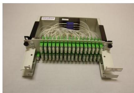
NC-1000 –monijaotinpaketti SC/APC
