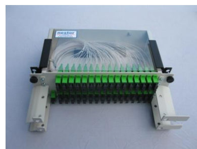
NC-1000 –jaotinmoduuli 1x64 SC/APC
