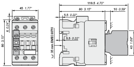
AF26, AF30, AF38 + CA4, CC4, 1-napainen apukosketinlohko
