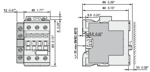
AF26, AF30, AF38 + CAL4-11, 2-napainen apukosketinlohko
