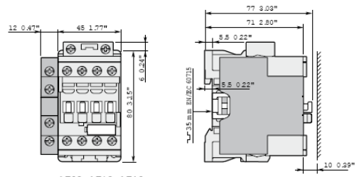
AF09, AF12, AF16 + CAL4-11, 2-napainen apukosketinlohko
