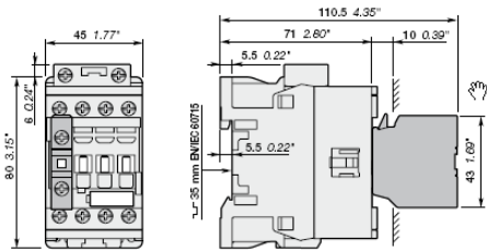
AF09, AF12, AF16 + CA4, CC4, 1-napainen apukosketinlohko
