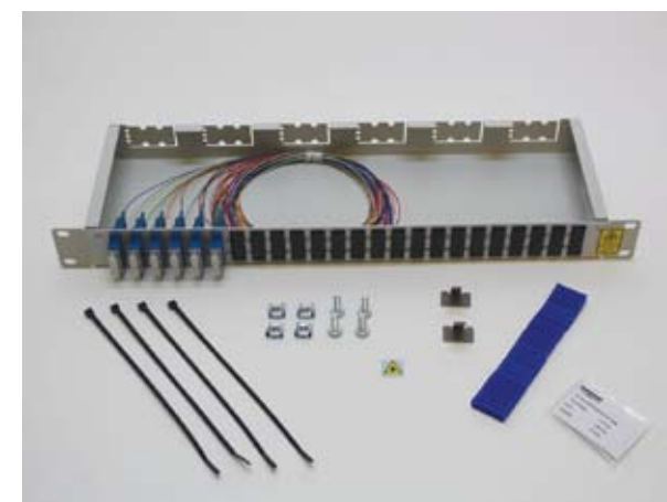
Vaihtoehtoinen päätepaneeli NC-230 esikalustettuna häntäkuitupakettina
