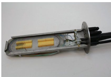
Jatkoskotelo NC-450 48-k asennettuna kaapelin kylkiotossa
