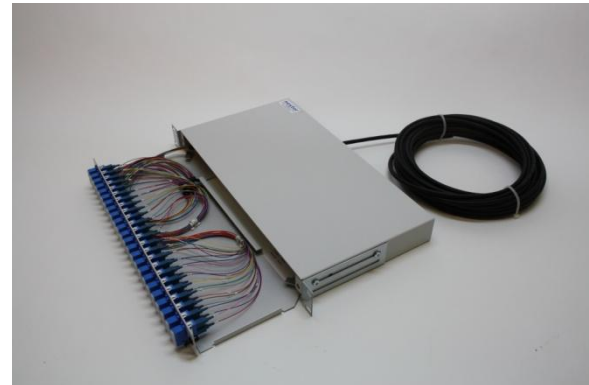
Päätepaneeli NC-200 häntäkuitu- ja häntäkaapelipakettina
