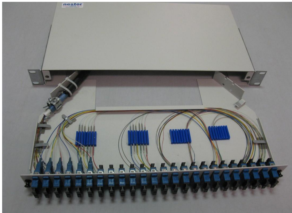
Päätepaneeli NC-200 asennettuna
