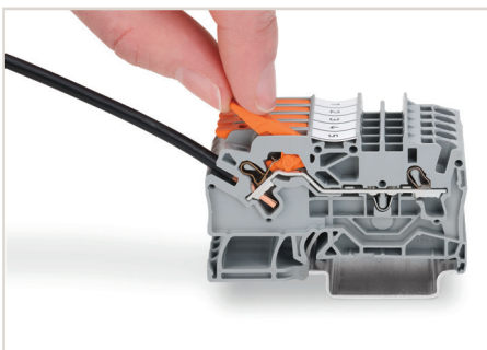
3. Sulje vipu.
