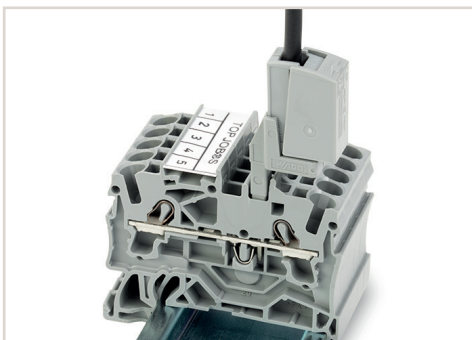
2009-182 mittausliitin käytännössä.
