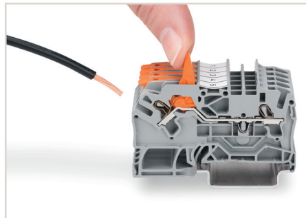
2. Avaa vipu - kytke.
