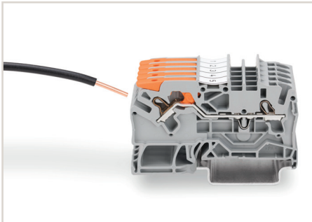
1. Helppokäyttöinen: jäykkä johdin voidaan kytkeä avaamatta vipua.
