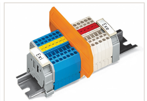
209-190 erotuslevy kiinnitettynä kiskoon.
