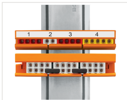
DIN-kiskoadapterilla kiinteä ja hyväksytty asennus.
