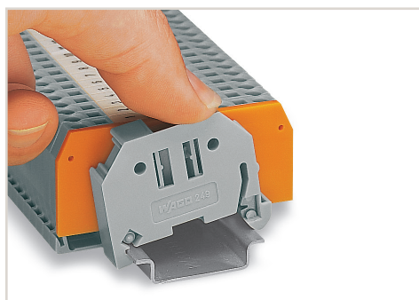
249-116 päätypuristin käytännössä.
